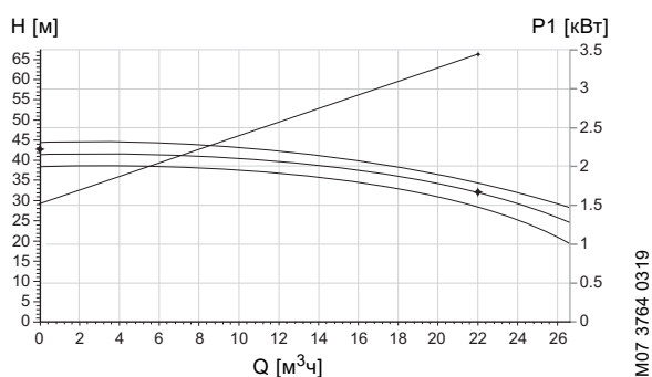
Рис. 96 Расчет значений на рис. 95 произведен для стандартной частоты вращения с целью сравнения с эталонной кривой рабочих характеристик
