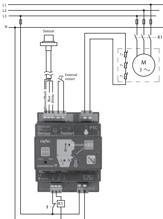
Рис. 70 Модуль LiqTec подключен к стандартному электродвигателю
