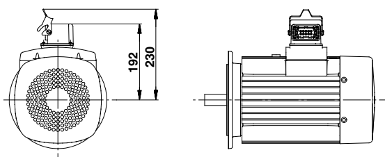
Рис. 19 Размеры, 1,5 - 7,5 кВт
