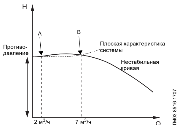
Рис. 111 Нестабильная кривая характеристик насоса
