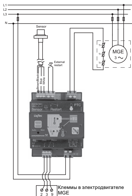
Рис. 72 Модуль LiqTec подключен к электродвигателю MGE (3-22 кВт)
