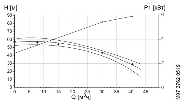
Рис. 98 Расчет значений на рис. 97 произведен для стандартной частоты вращения с целью сравнения с эталонной кривой рабочих характеристик
