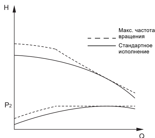
Рис. 110 Кривая рабочих характеристик стандартного электродвигателя (60 Гц) по сравнению с кривой рабочих характеристик насоса, работающего с максимальной частотой вращения.
