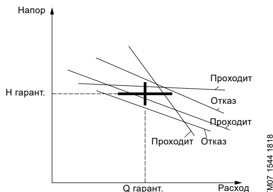
Рис. 93 Кривые насоса, которые проходят через допустимую область гарантируемой точки или не попадают в нее
