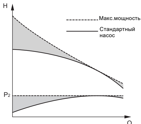
Рис. 108 Кривые характеристик стандартного E-насоса и насоса, работающего на пределе мощности
