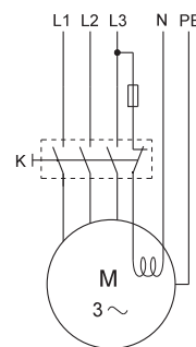
Рис. 25 Трехфазный электродвигатель с антиконденсатным нагревателем
