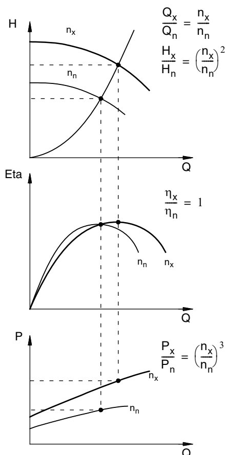
Рис. 106 Уравнения подобия
