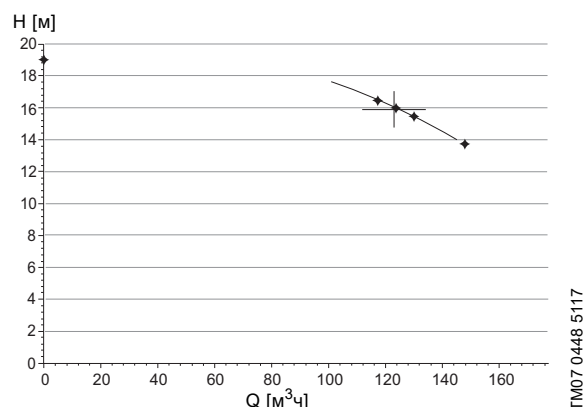
Рис. 92 Для определения одной гарантируемой точки используются результаты замеров на пяти контрольных точках
