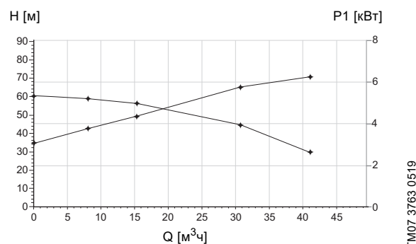
Рис. 97 Результаты измерений для испытываемого насоса
