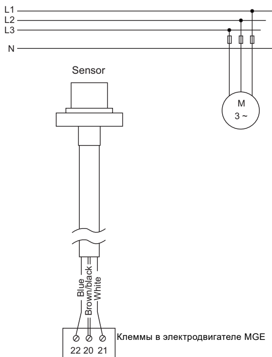
Рис. 71 Модуль LiqTec подключен к электродвигателю MGE (0,37 - 2,2 кВт)
