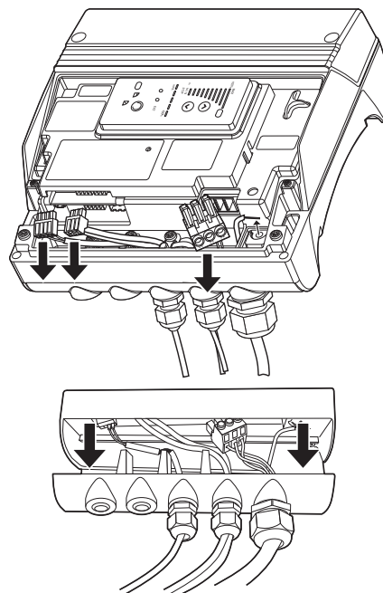
Рис. 23 Расположение съемной кабельной планки на клеммной колодке электродвигателя, а также соединители для подключения электросети, датчика и интерфейса связи.
