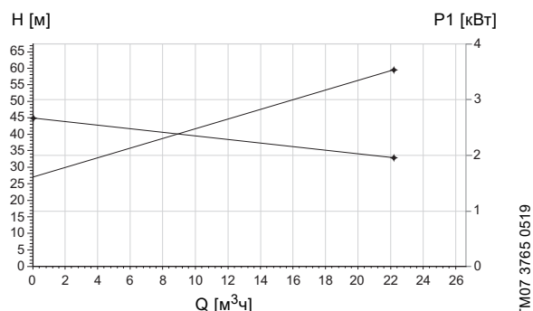
Рис. 95 Результаты измерений для испытываемого насоса
