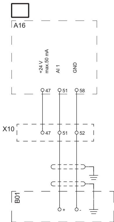
Сигнал потока
