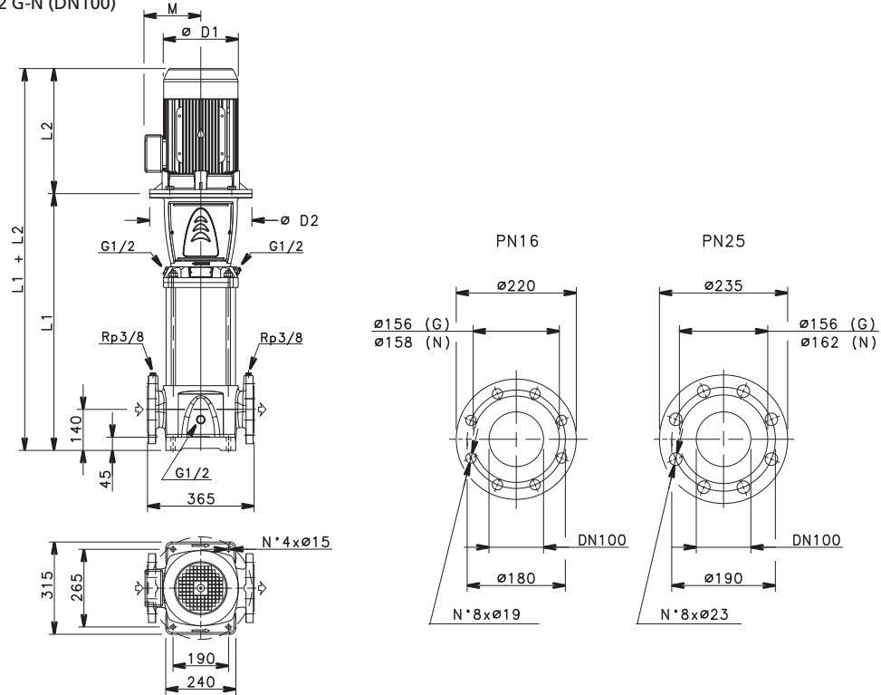
100-92 G-N (DN100)
